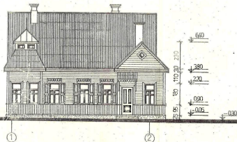
FASADAS 1-2 M1:100
